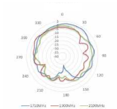
1710-2100MHz
