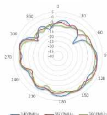
3400-3800 MHz
