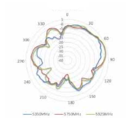
5350-5925 MHz
