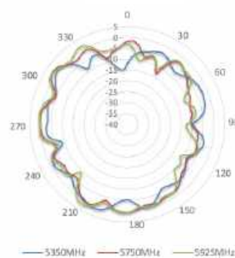
5350-5925 MHz
