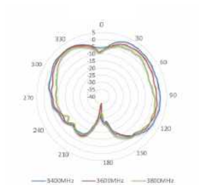
3400-3800 MHz
